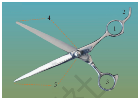
图 1-1-22 美容剪的结构
